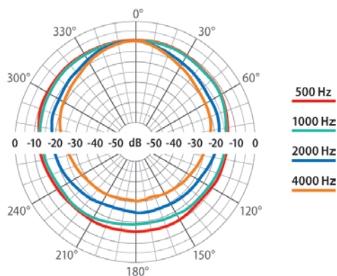
Kruhový diagram smerovej charakteristiky:
