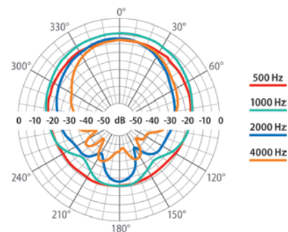
Kruhový diagram smerovej charakteristiky – vertikálne:
